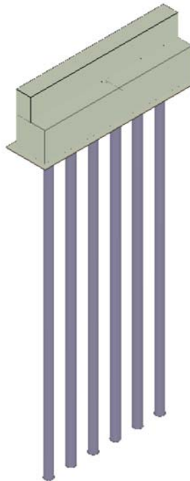
Figura 1 - Vista assonometrica
